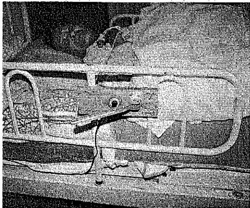
ナースコール改良タイプA
